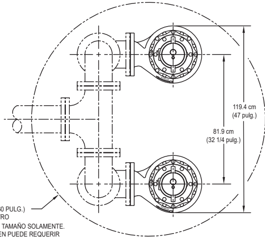
INSTALACIÓN DÚPLEX
