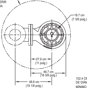
INSTALACIÓN SIMPLEX
