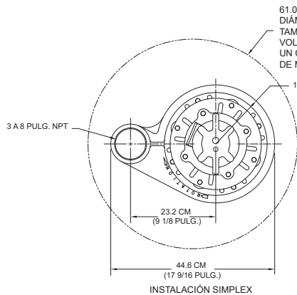
INSTALACIÓN SIMPLEX
