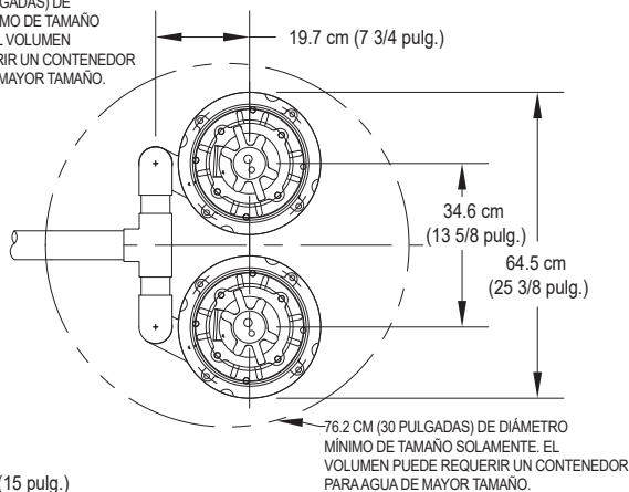
INSTALACIÓN DÚPLEX
