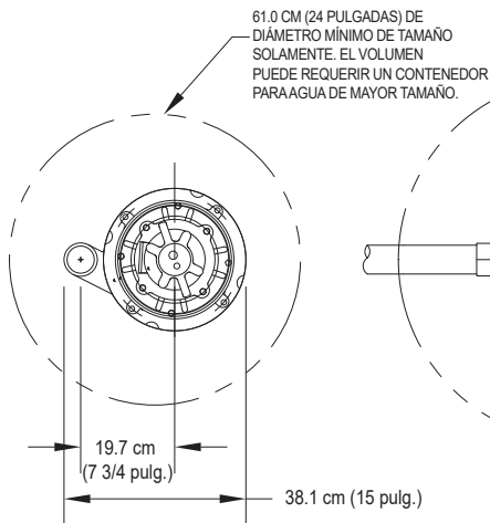
INSTALACIÓN SIMPLEX
