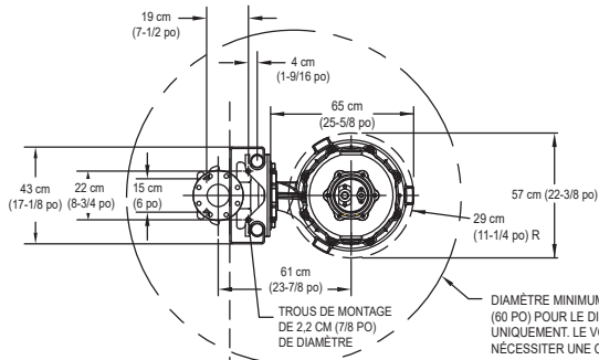
PLAN DE RÉF. CADRE DE LA PORTE
