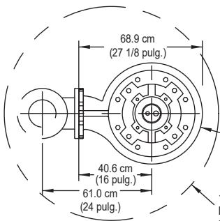
INSTALACIÓN SIMPLEX
